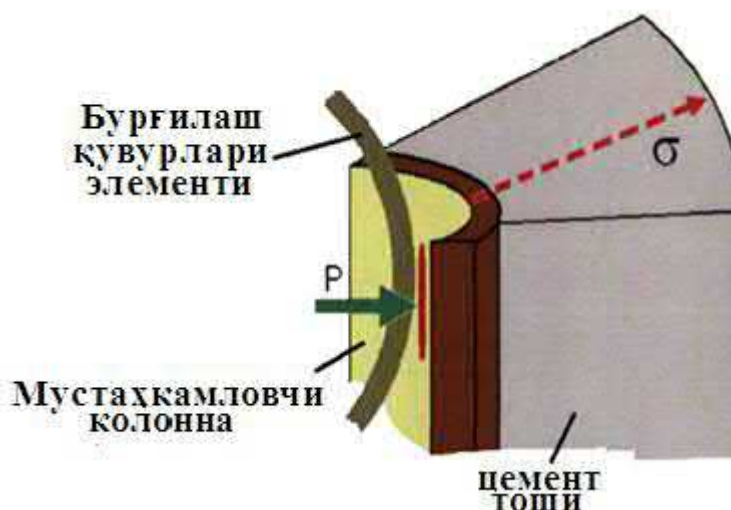
3-расм. Қудукни чуқурлаштириш жараёнида босим ва нормал кучланишнинг тарқалиши диаграммаси:
